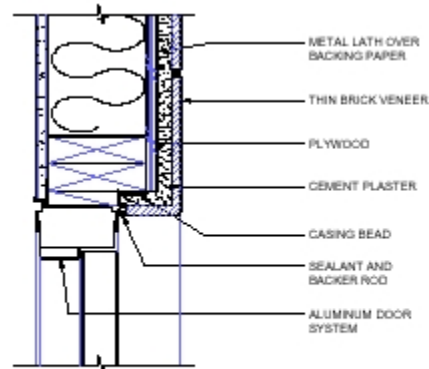
DOOR JAMB
