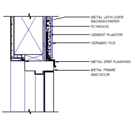
DOOR HEAD
