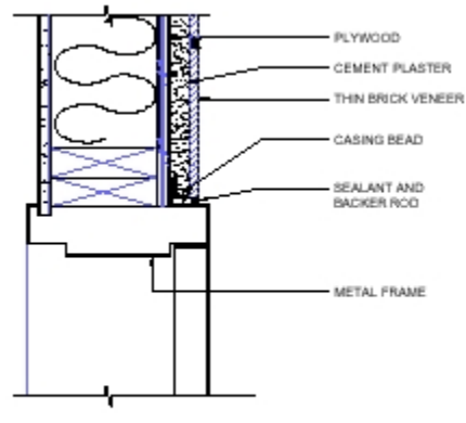
DOOR JAMB
